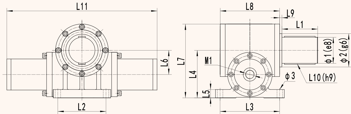
BJZD 脚架式轴输出单齿条系列摆动油缸
