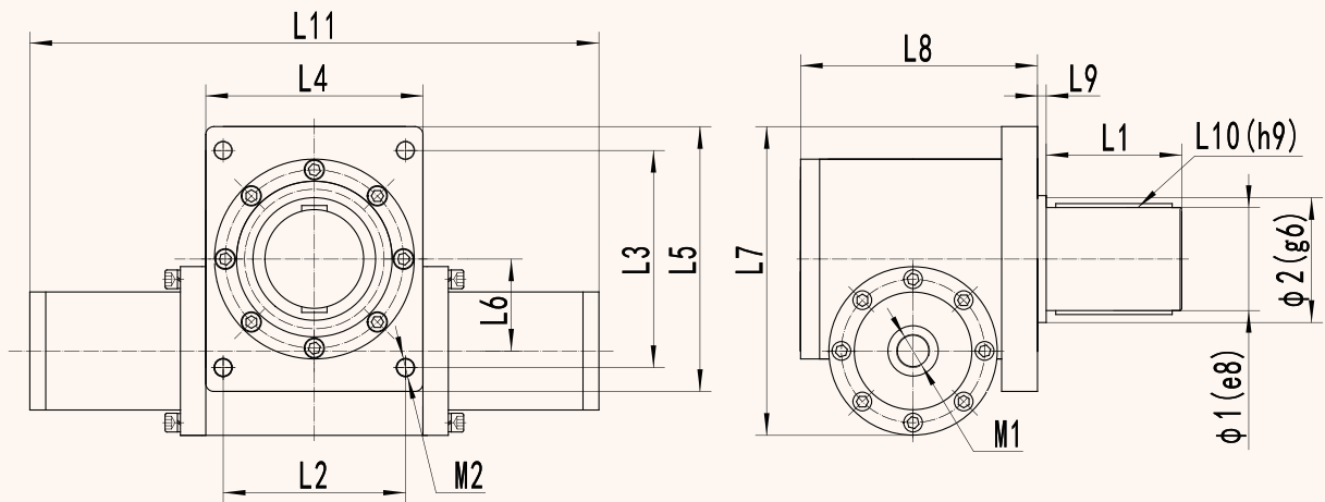
BFZD 法兰式输出单齿条系列摆动油缸
