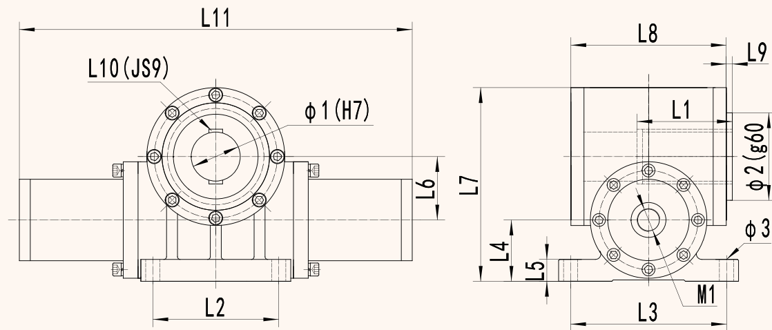
BJKD 脚架式孔输出单齿条摆动油缸外形尺寸
