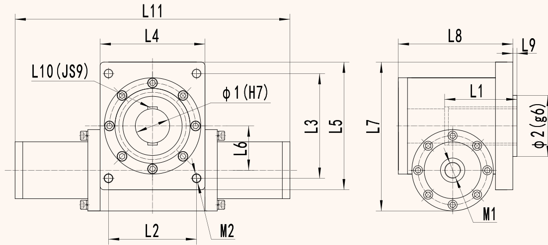
BFKD 法兰式孔输出单齿条摆动油缸外形尺寸
