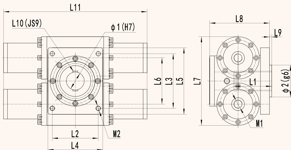
BFKS 法兰式孔输出双齿条摆动油缸外形尺寸
