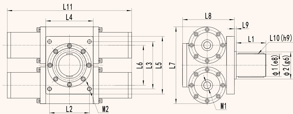
BFZS 法兰式轴输出双齿条摆动油缸外形尺寸
